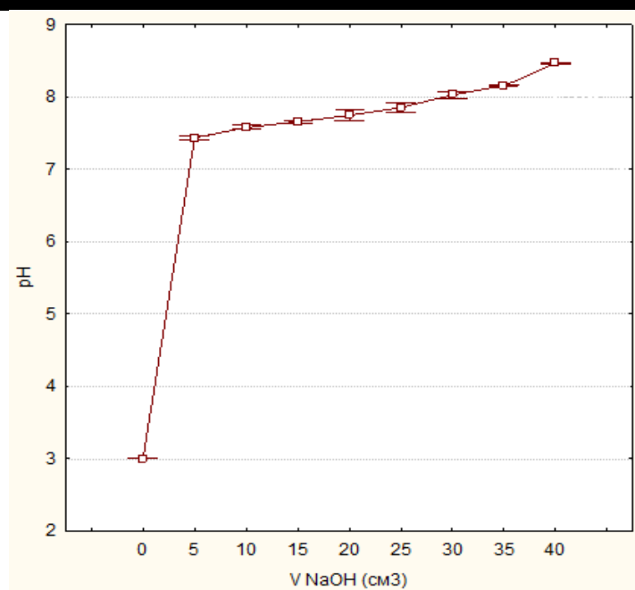
Рисунок 1 – Кривая потенциметрического титрования донных отложений раствором 0,1 м NaOH (доза \text{Ni}^{2+} 3 ПДК)
