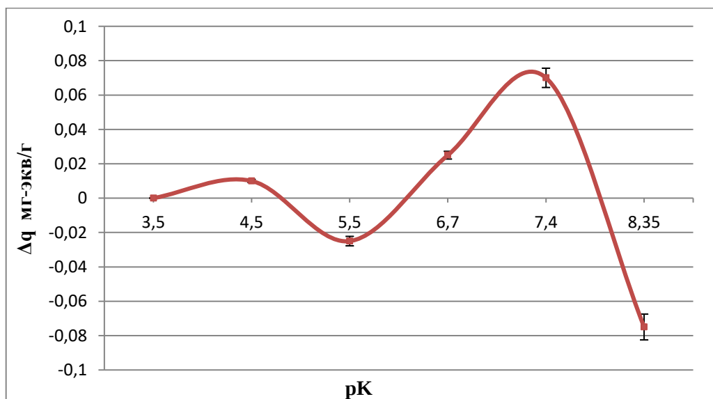
Рисунок 2 – Зависимость приращения протолитической емкости донных отложений от значений рК функциональных групп (доза \text{Ni}^{2+} 3 ПДК)
